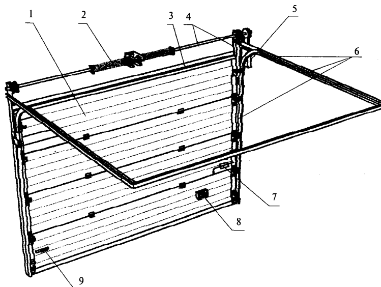
Рисунок А.3 — Пример конструкции подъемно-поворотных ворот
