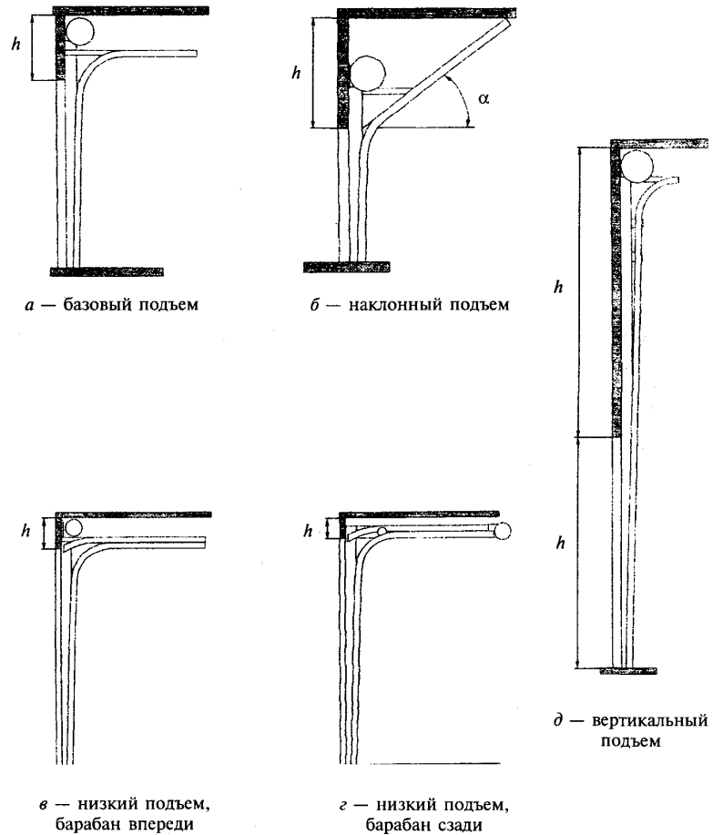
Рисунок А.5 — Схемы вариантов подъемов подъемно-секционных ворот
