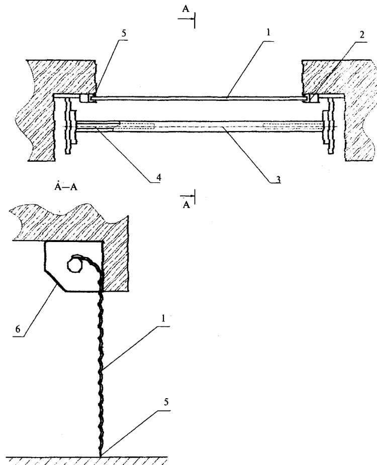
Рисунок А.7 — Пример конструкции складывающихся ворот
