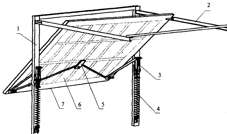
Рисунок А.2 — Пример конструкции откатных ворот с нижней опорной балкой
