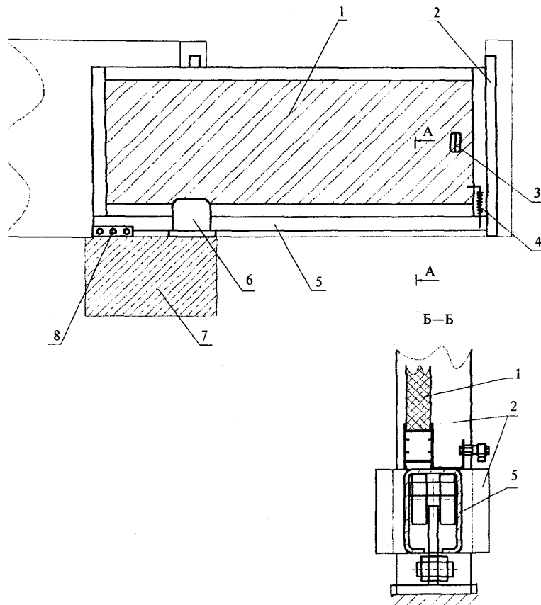
Рисунок А.1 — Пример конструкции распашных ворот с утепленным щитовым полотном
