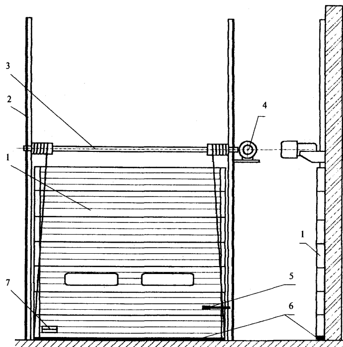
1 — полотно ворот; 2 — направляющие профили; 3 — система уравновешивания полотна; 4 — привод; 5 — задвижка; 6 — уплотнители; 7 — ручка
